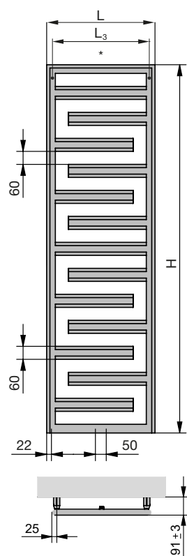
Teplovodní provoz: středové připojení
