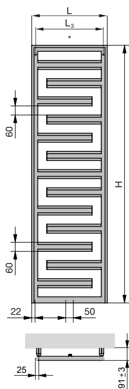
Teplovodní provoz: vnější připojení
